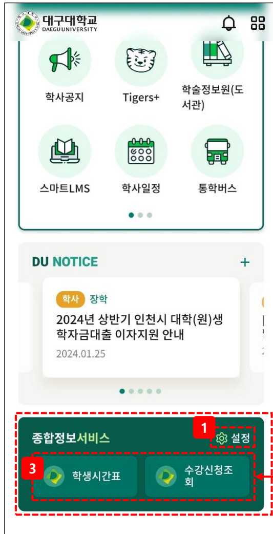
홈 - 종합정보서비스
