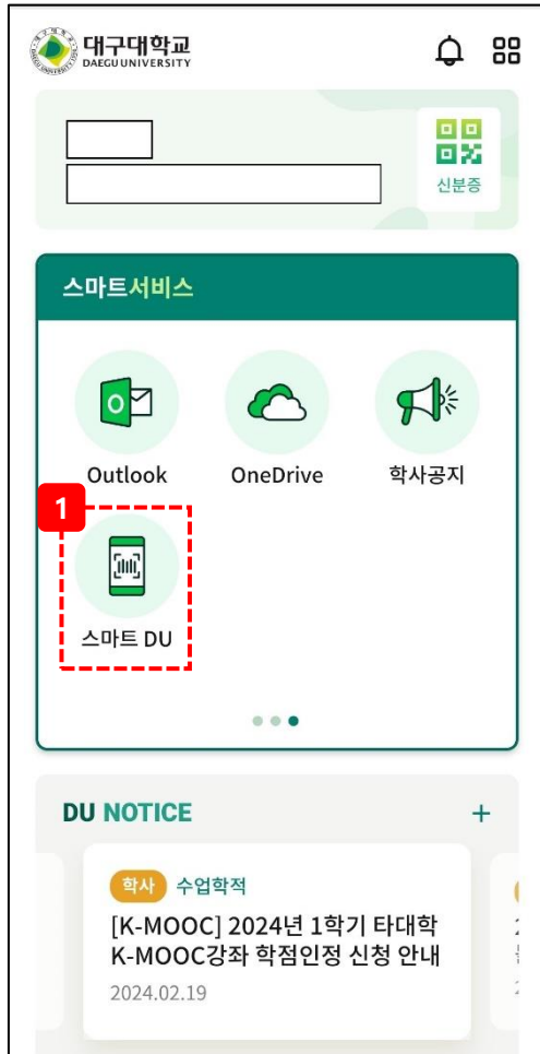
스마트 DU
