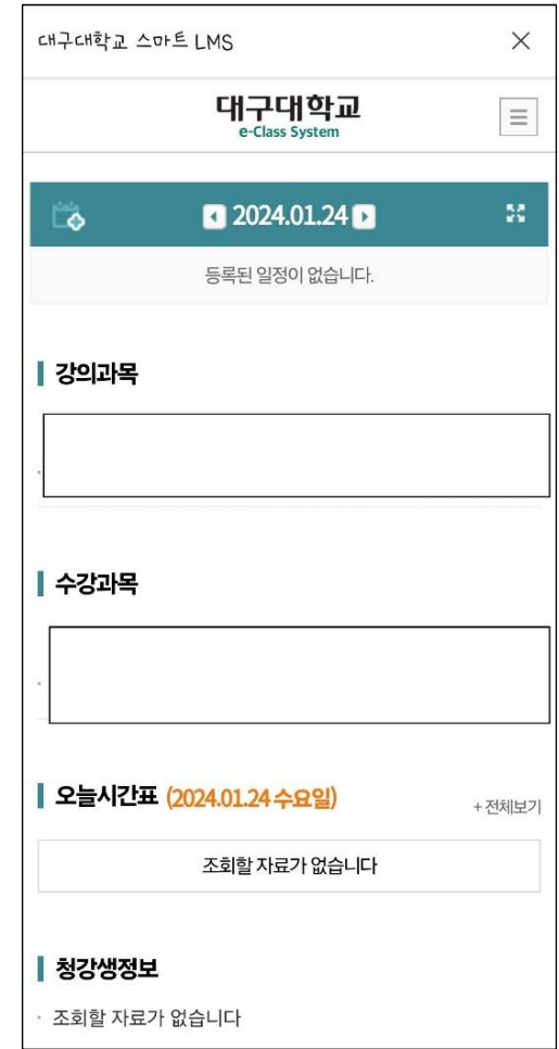
스마트 LMS
