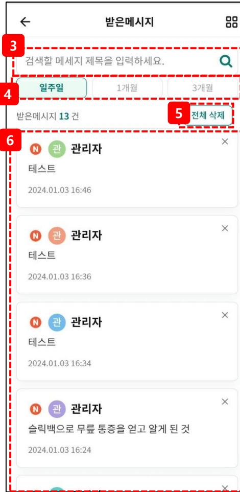
받은 메시지
